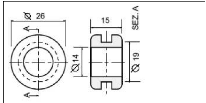
ART. N°002518
