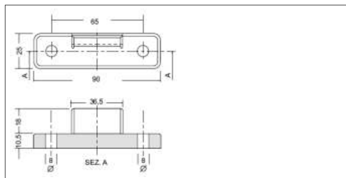
ART. N°1039-S
